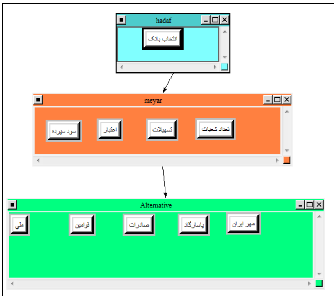
شکل ۱: مدل AHP مساله
